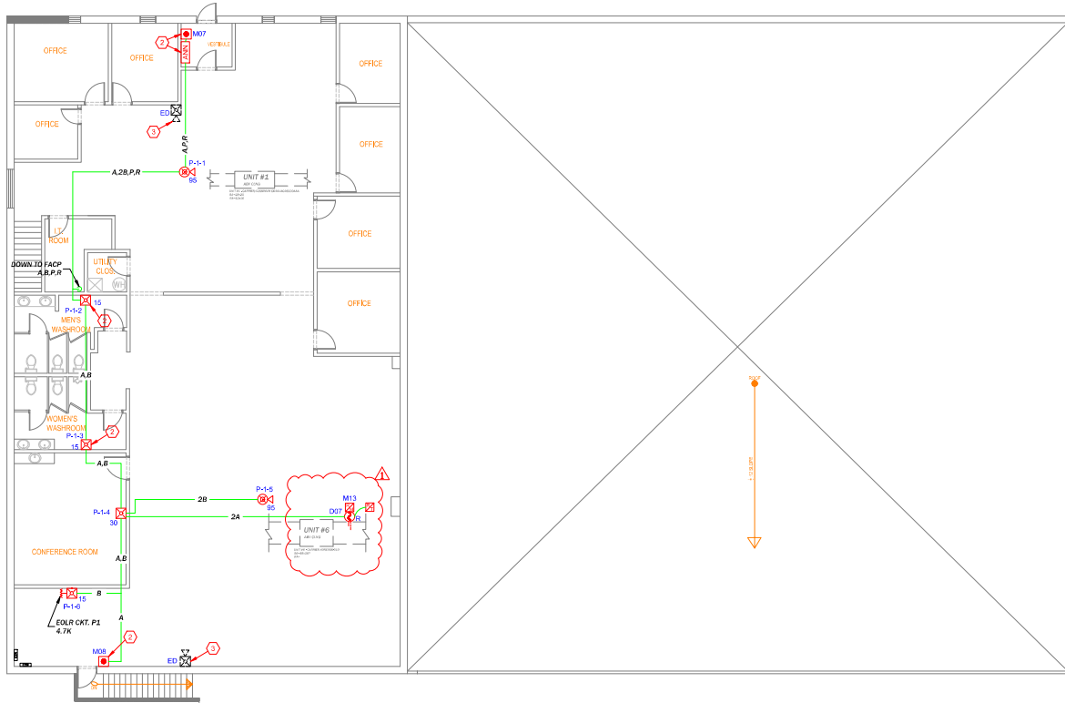
1 UPPER LEVEL - FIRE ALARM PLAN SCALE: 1/8" = 1'-0" 2' 0' 4' 8' SCALE: 1/8" = 1'-0"
