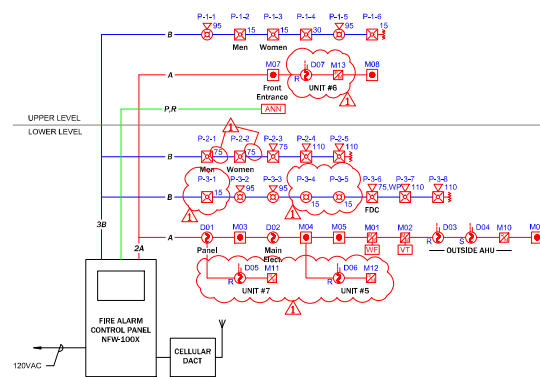
2 RISER DIAGRAM SCALE: NONE
